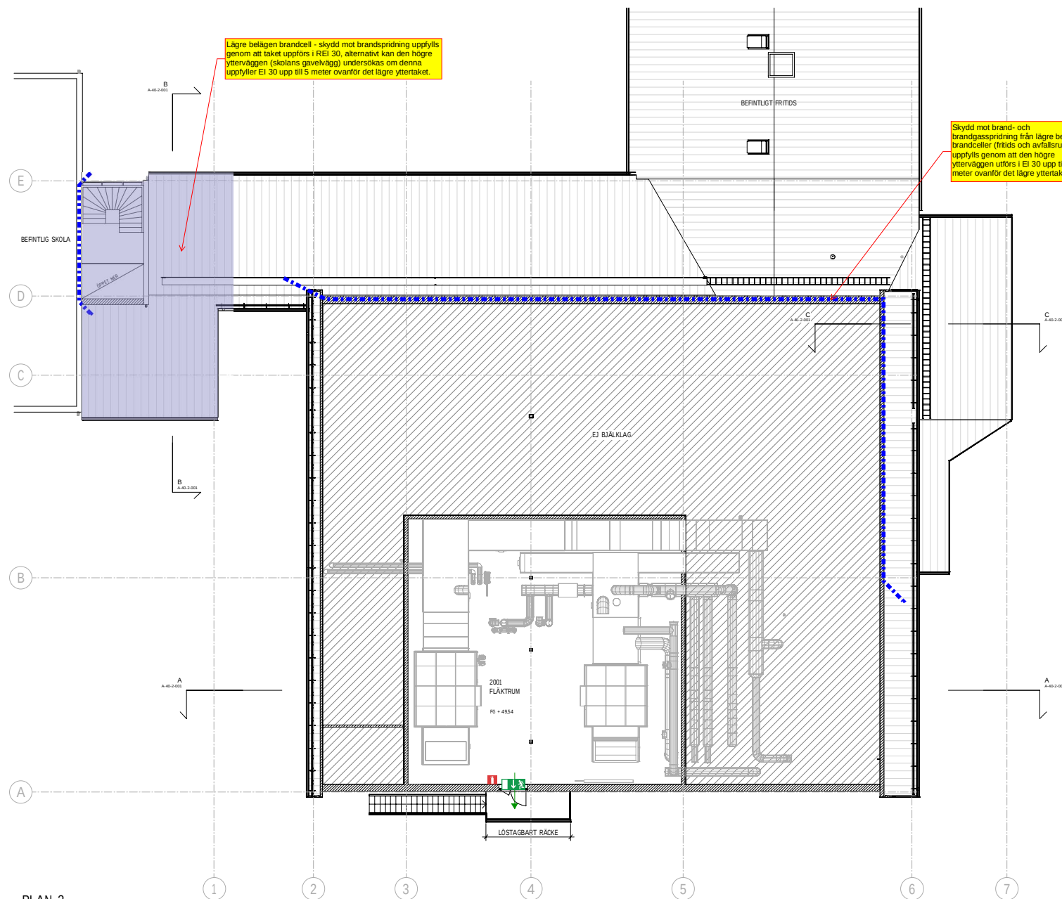
PLAN 2 1 : 100
